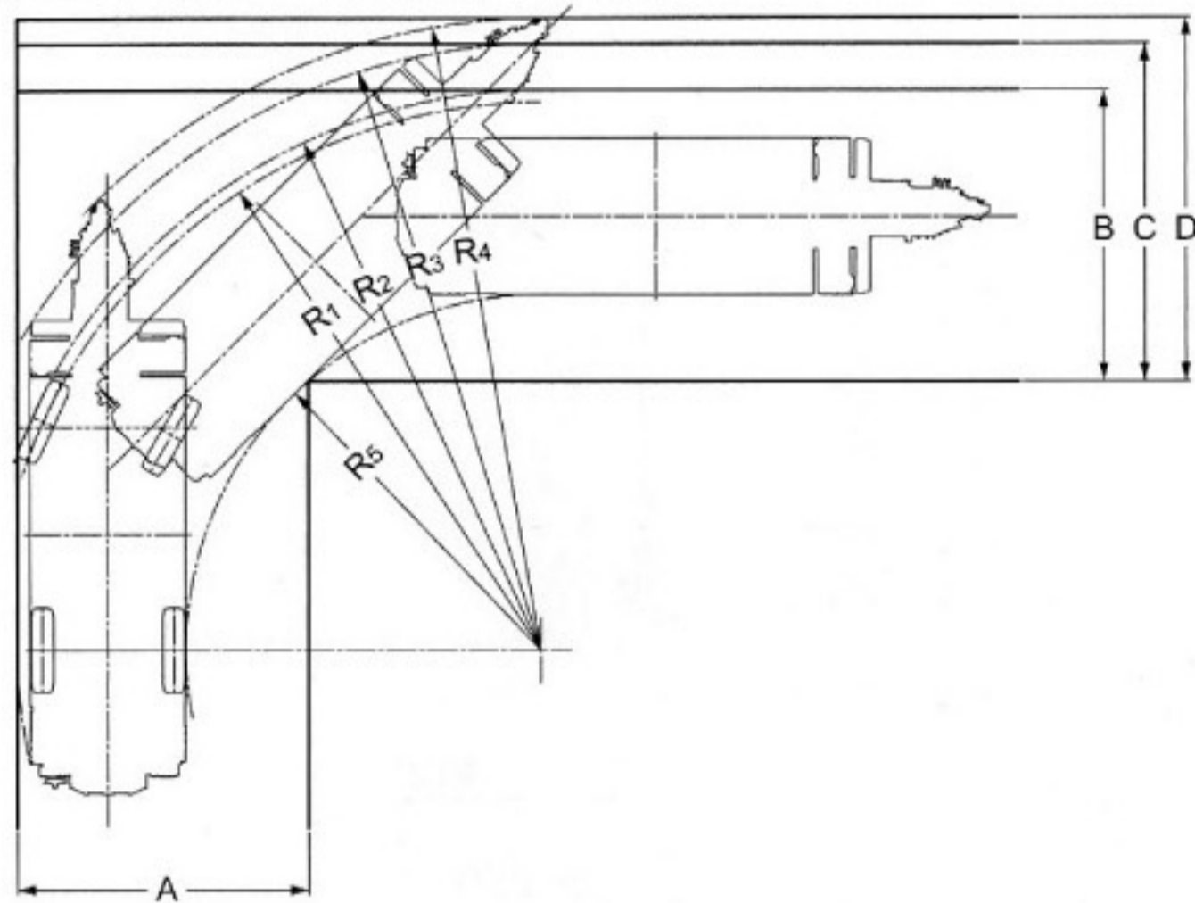
●2輪ステアリングで右折する場合
