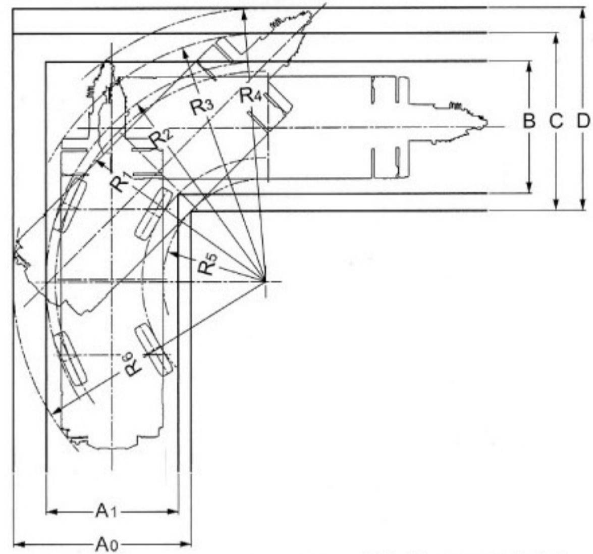
●4輪ステアリングで右折する場合
